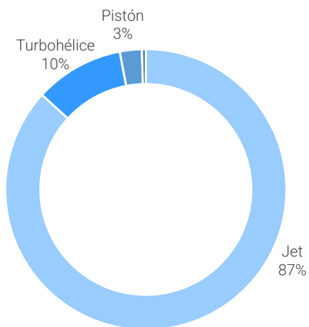
% Aeronaves por Tipo de Motor
