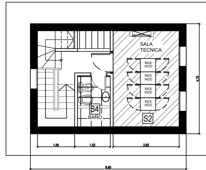
PLANTA 3° PISO
