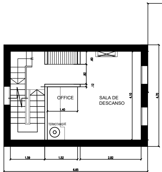
PLANTA 2° PISO
