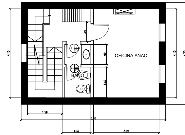
PLANTA 1° PISO
