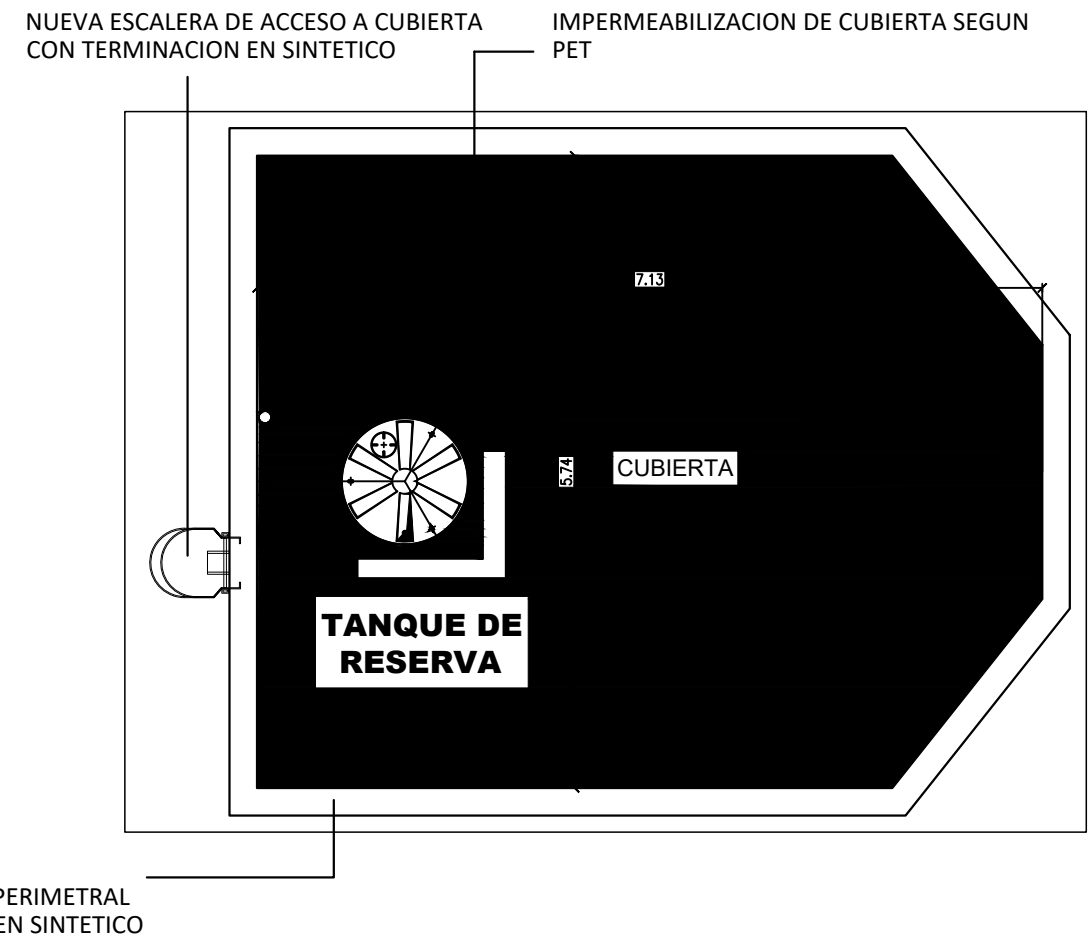
PLANTA CUBIERTA
