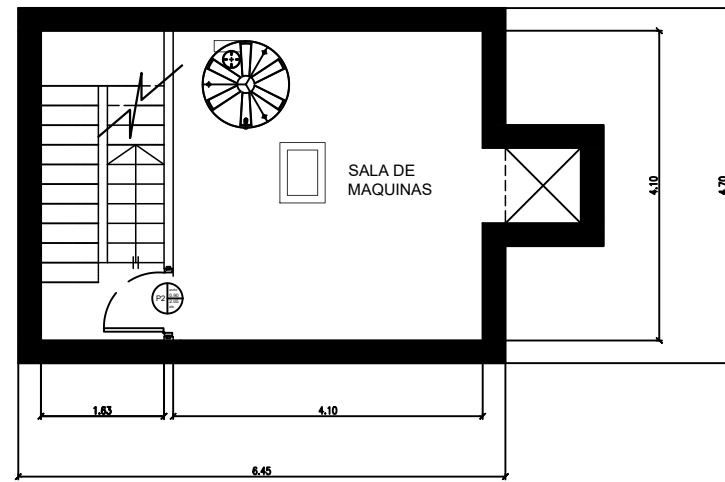
PLANTA SUBSUELO
