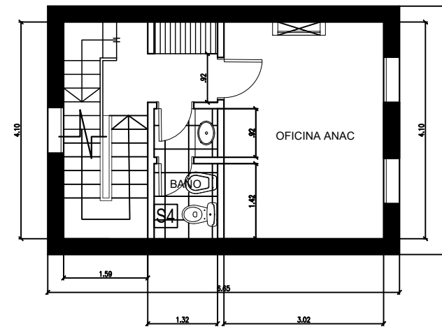
PLANTA 1° PISO
