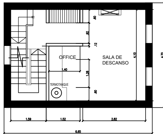
PLANTA 2° PISO
