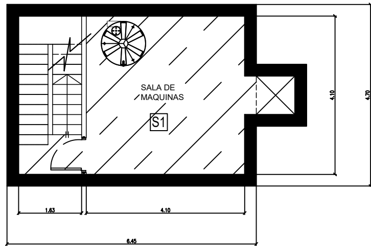
PLANTA SUBSUELO
