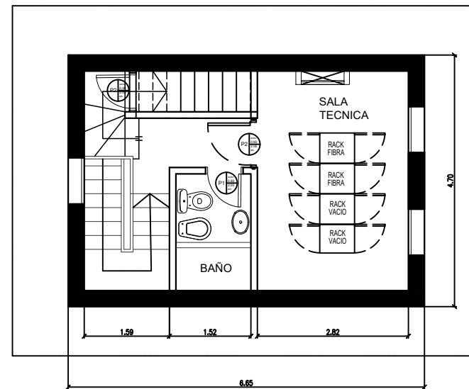
PLANTA 3° PISO
