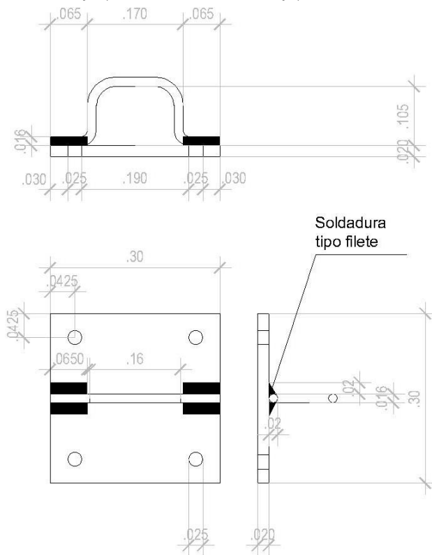
A modo de ejemplo. Placas metálicas de anclaje para arriostamiento de TWR FAA
